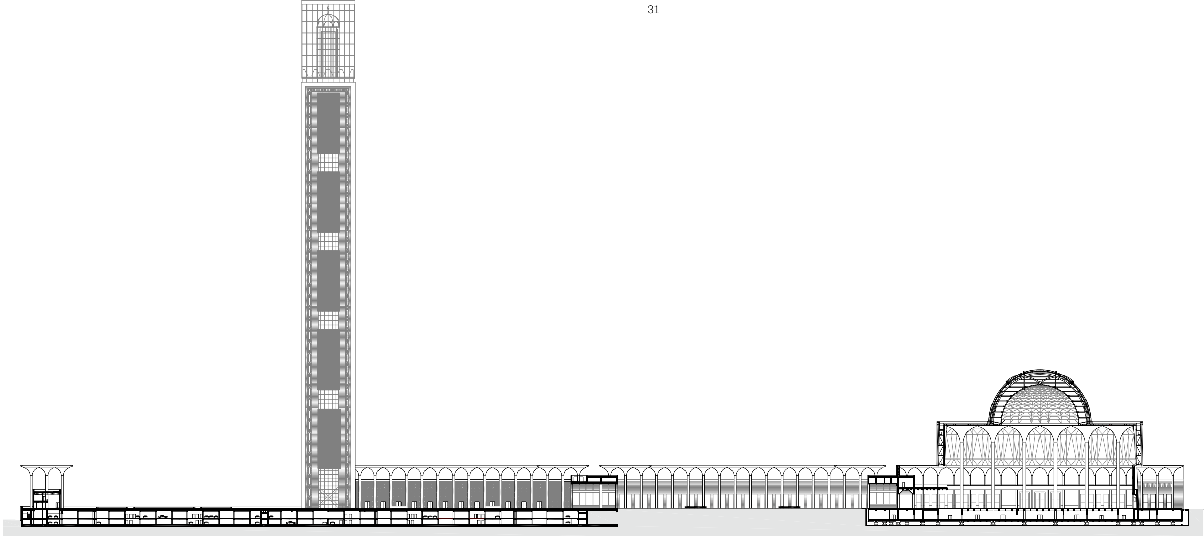
Schnitt Section
