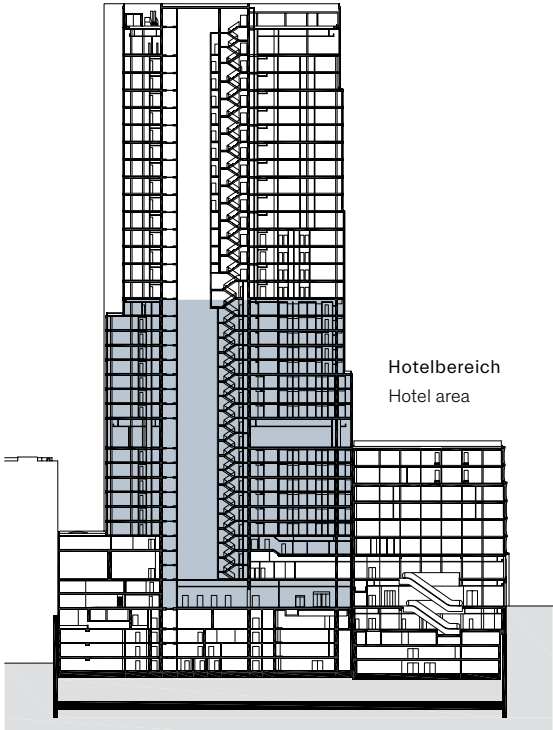
Schnitt Section
