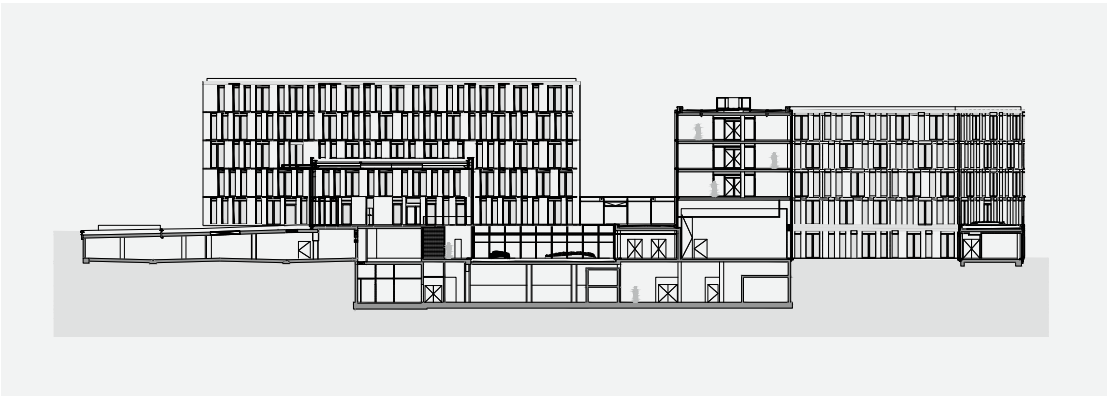
Schnitt Section
